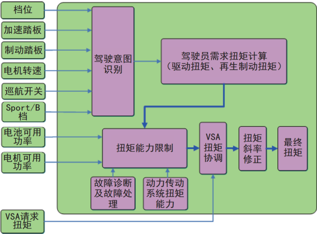
VCU 整车控制动力系统行驶控制图
